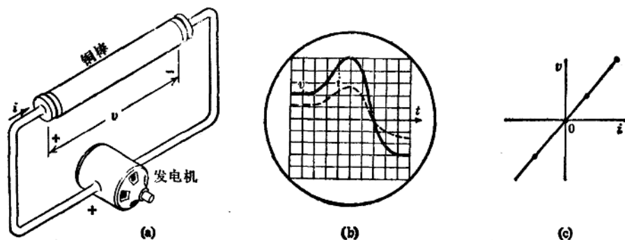
图 1.4 确定电阻器特性的实验
