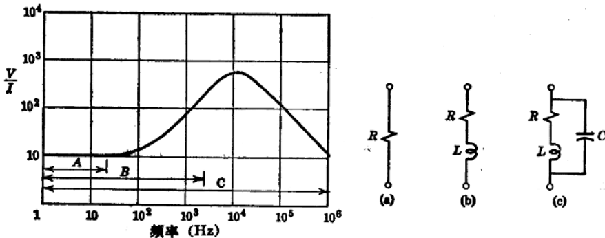
图 1.1 线圈特性和电路模型
