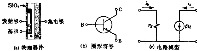
图 1.2 晶体管表示法
