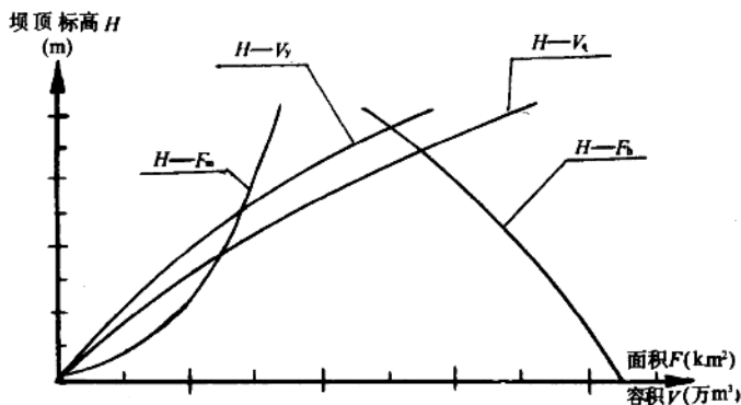
图 2-6 尾矿库性能曲线
