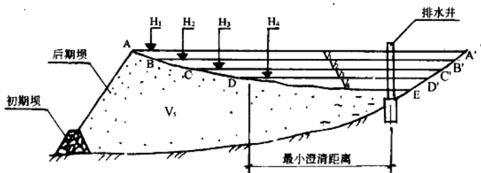
图 2-5 尾矿库库容组成示意图
