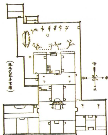
浙江藏书楼平面图
