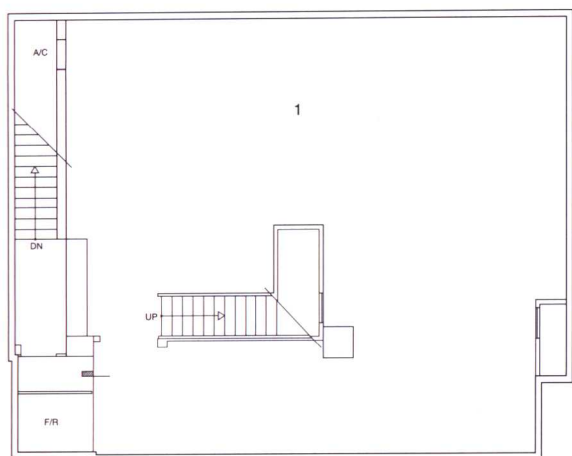
地下一层平面图 1- 展示室
