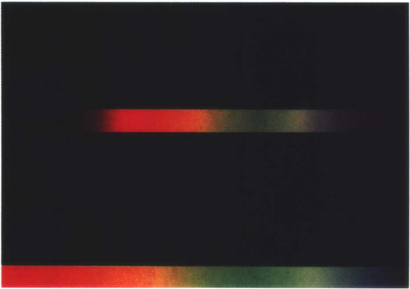
(特征光谱)
