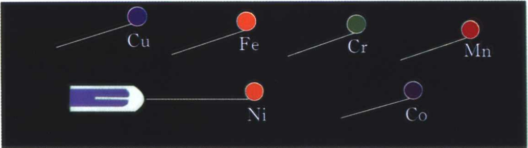
(硼砂珠反应)
