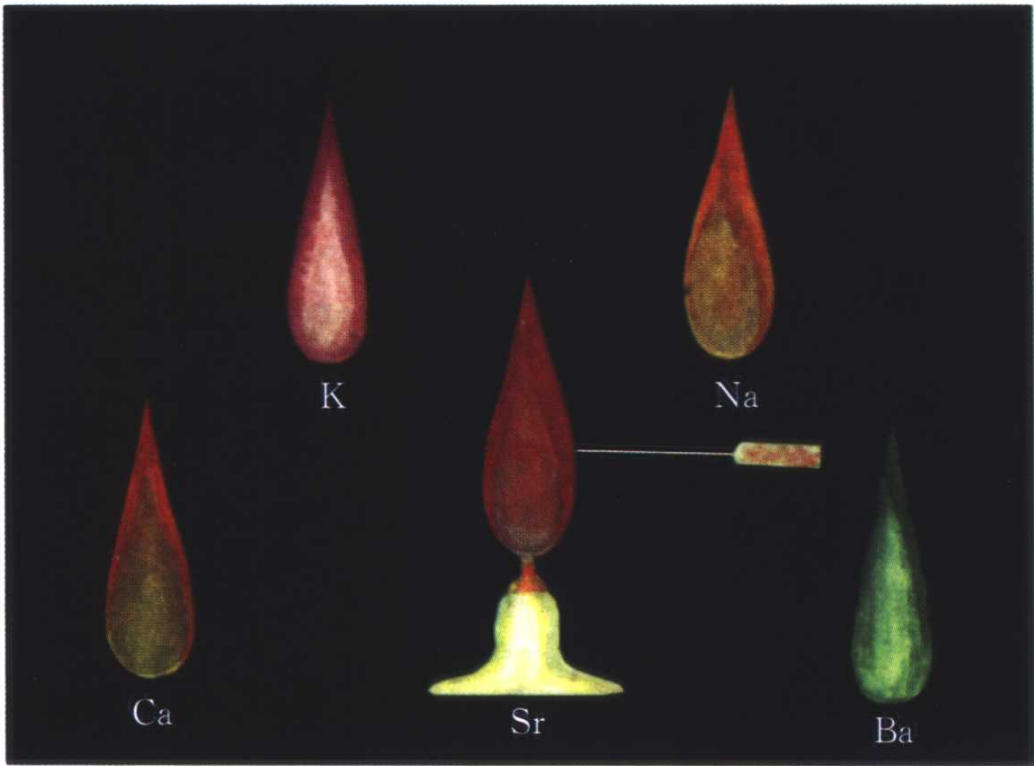
(焰色反应)
