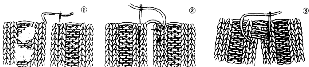
双罗纹缝合
