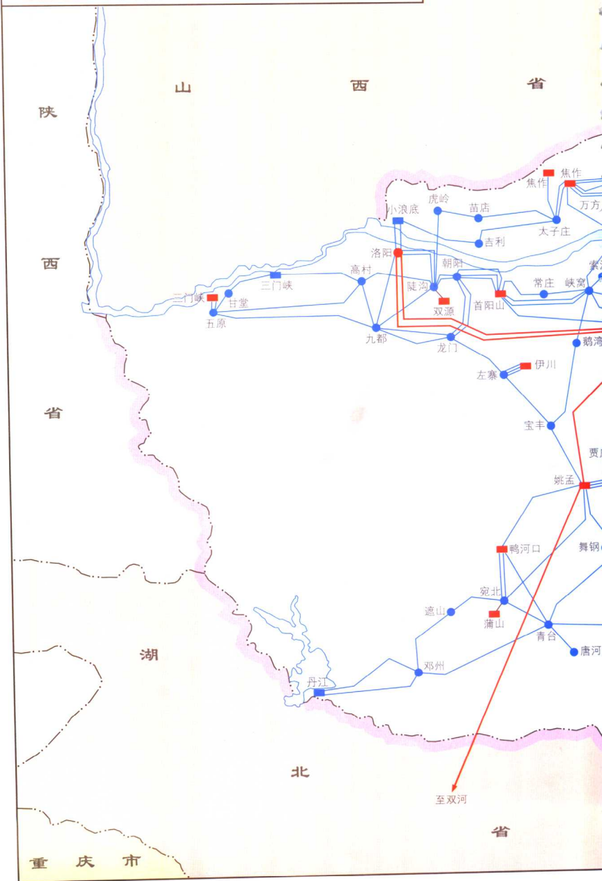
一九九九年河南电网地理位置接线示意图
