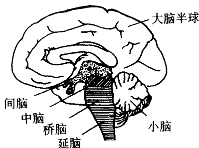
图 4 人脑各部位
