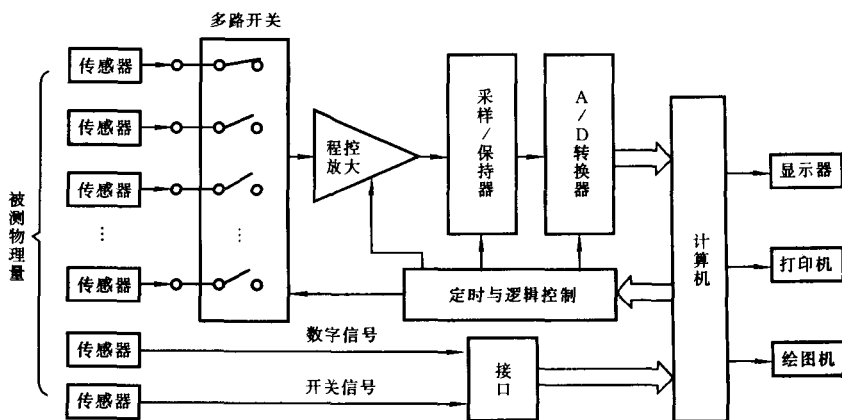
图 1-1 微型计算机数据采集系统框图
