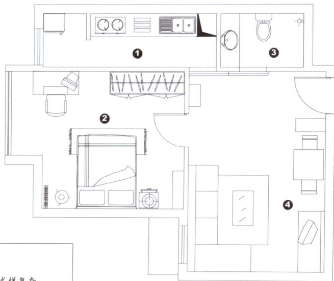
平面布置图
