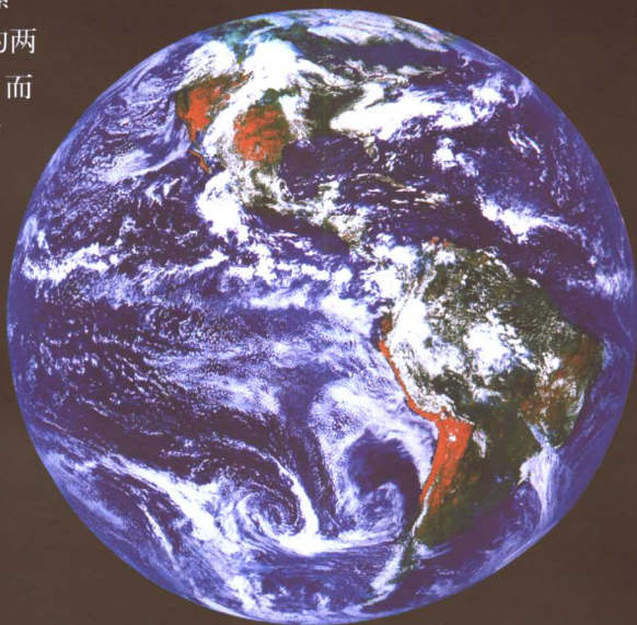
■ 这张照片是由安装在气象卫星上的照相机在赤道上空35800千米的高空拍摄的,当时卫星正飞过美洲上空。它显示了深蓝色的海洋和大气中翻卷的云层,这都是适合生命存在的必要条件。
