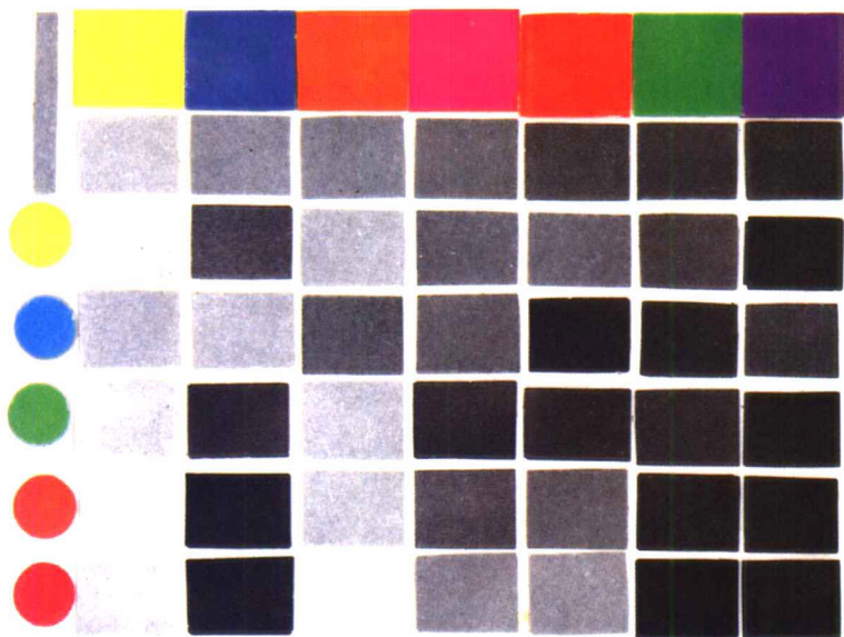
图7 摄影色标（加用滤色镜）（灰条表示未加色镜各色在黑白照片上所呈灰阶，各圆点表示加用黄、蓝、绿黄、橙、红色镜后各色在黑白照片上所呈灰阶）
