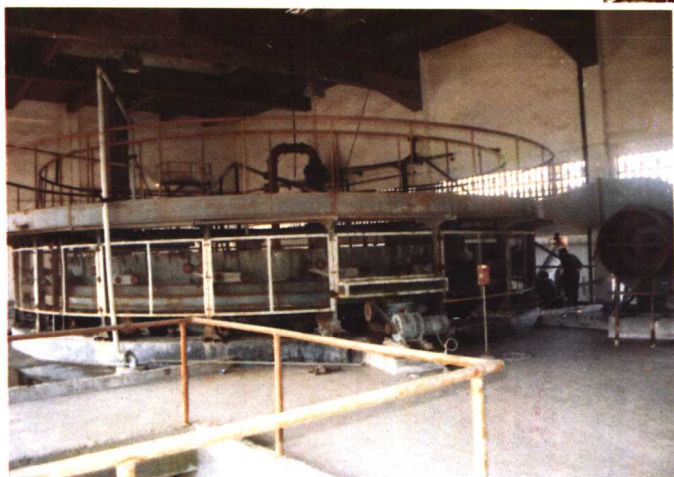
龙海磷肥厂3万吨/年磷铵车间园盘过滤机
