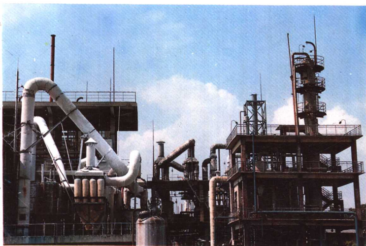
福州第二化工厂聚氯乙烯汽提干燥系统
