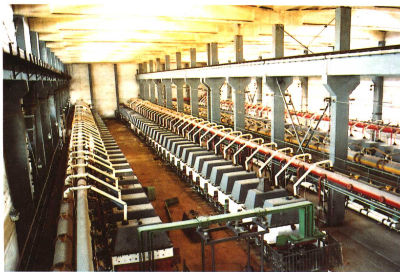
福州第二化工厂烧碱车间金属阳极电解槽
