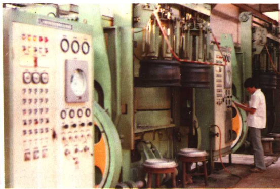
邵武轮胎厂外胎自动定型硫化装置
