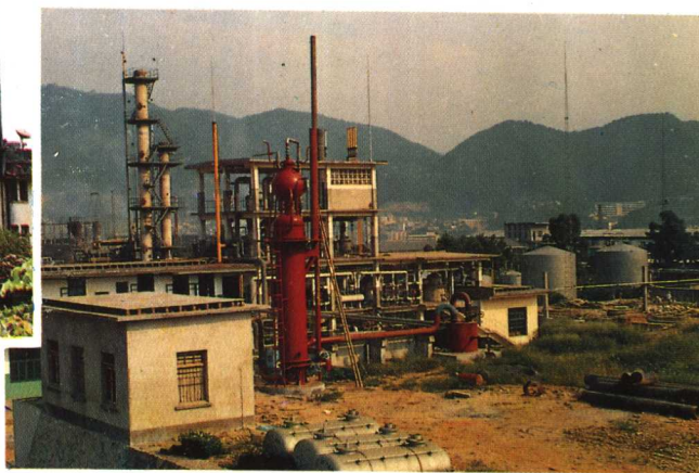
三明化工总厂甲醛生产装置
