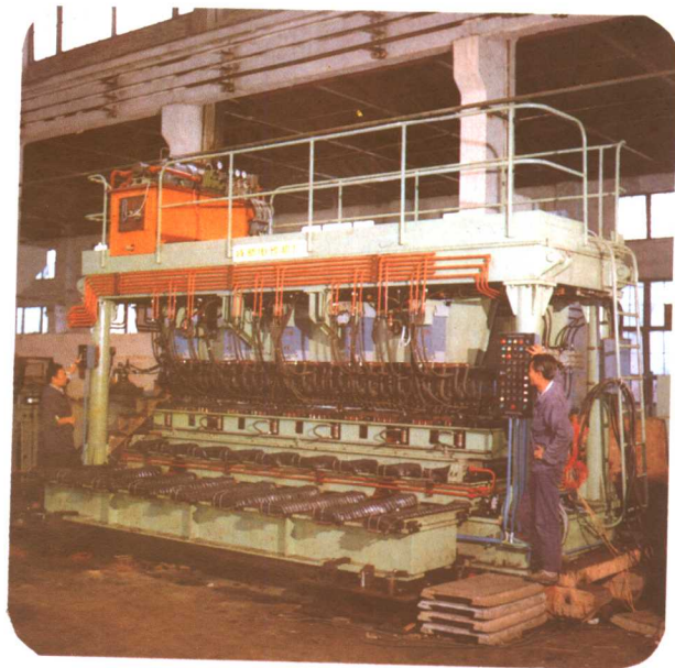
汽车多点焊机
