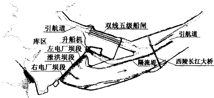
图 1-1 三峡水利枢纽平面布置简图
