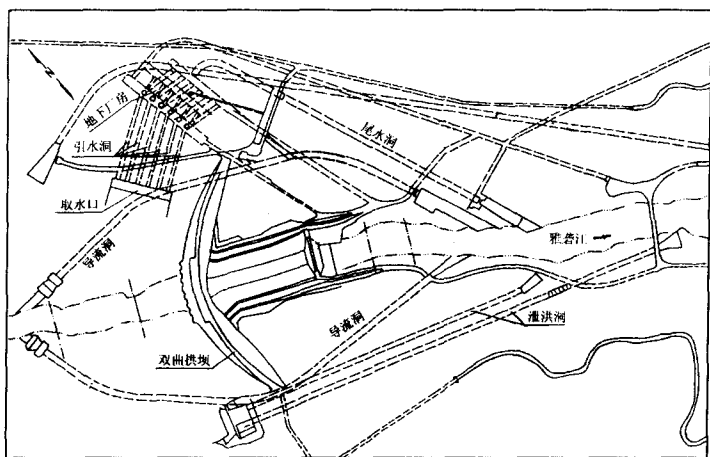
图 1-2 二滩水电站水利枢纽布置图
