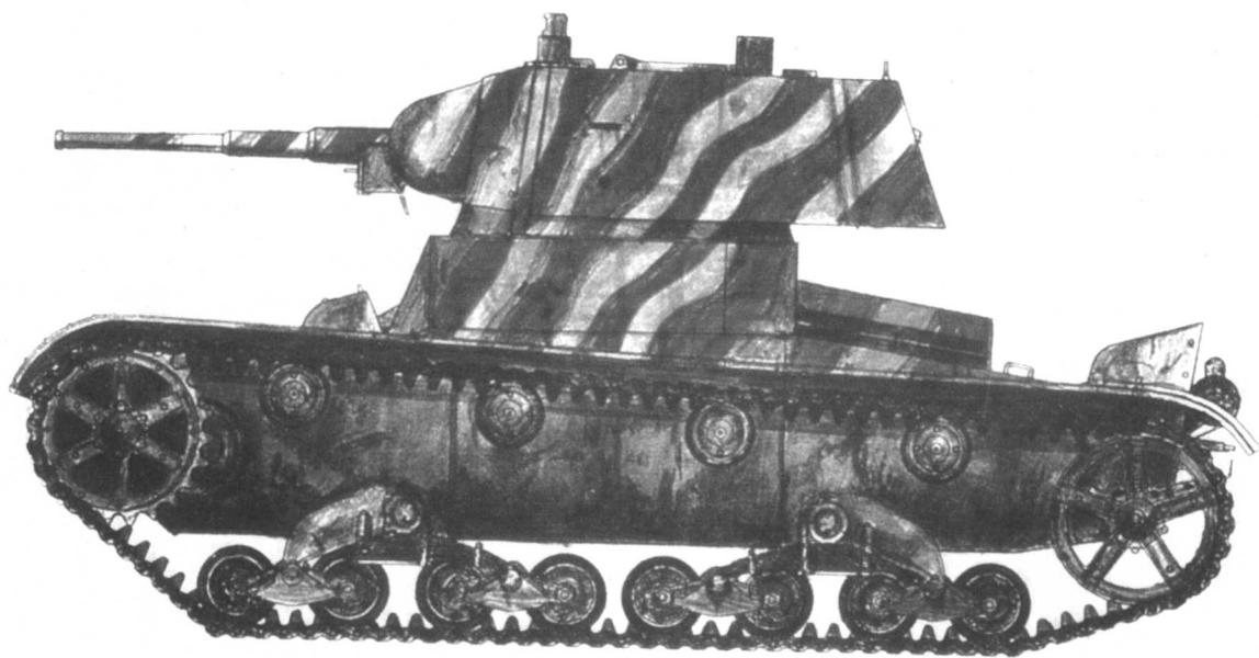
前苏联 1941 年 6-7 月，西部前线的 T-26S(1939 年型)轻型坦克
