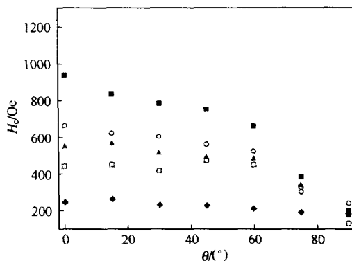
图 1-7 不同直径但长径比均为 50 的 Ni 纳米线阵列的矫顽力 H_c 与外加磁场方向和多孔氧化铝表面的法线之间的夹角 \theta 的依赖关系 直径分别为: ■ 18nm; ○ 10nm; ▲ 9nm; □ 8nm; ◆ 7nm
