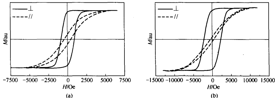
图1-2 Ni纳米线阵列的磁滞回线(a)和Fe纳米线阵列的磁滞回线(b)
