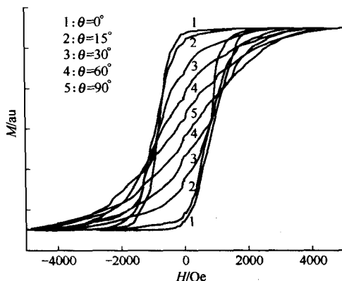
图 1-5 Ni 纳米线阵列的磁滞回线
