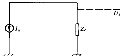
图 2.4 共阻抗系统
