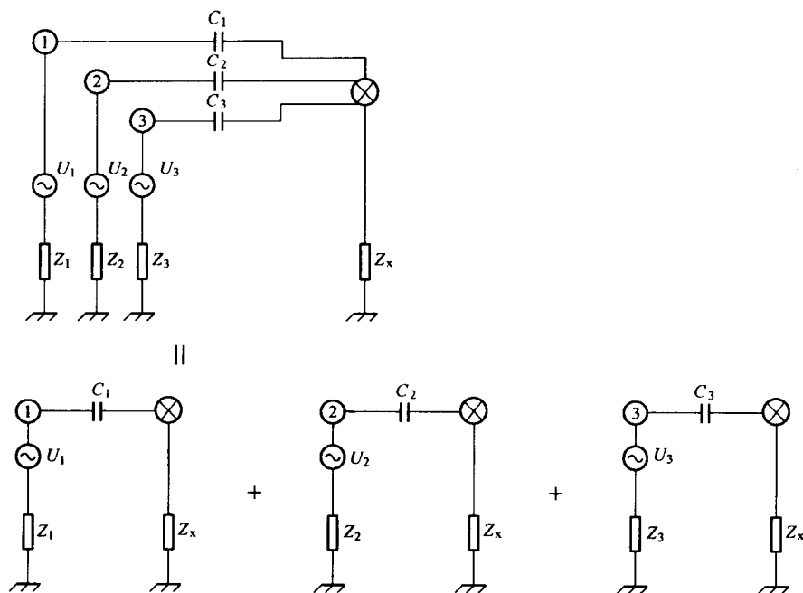
图 2.2 由若干干扰源引起的干扰电压
