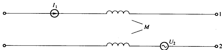
图 2.3 邻近导线的电磁耦合
