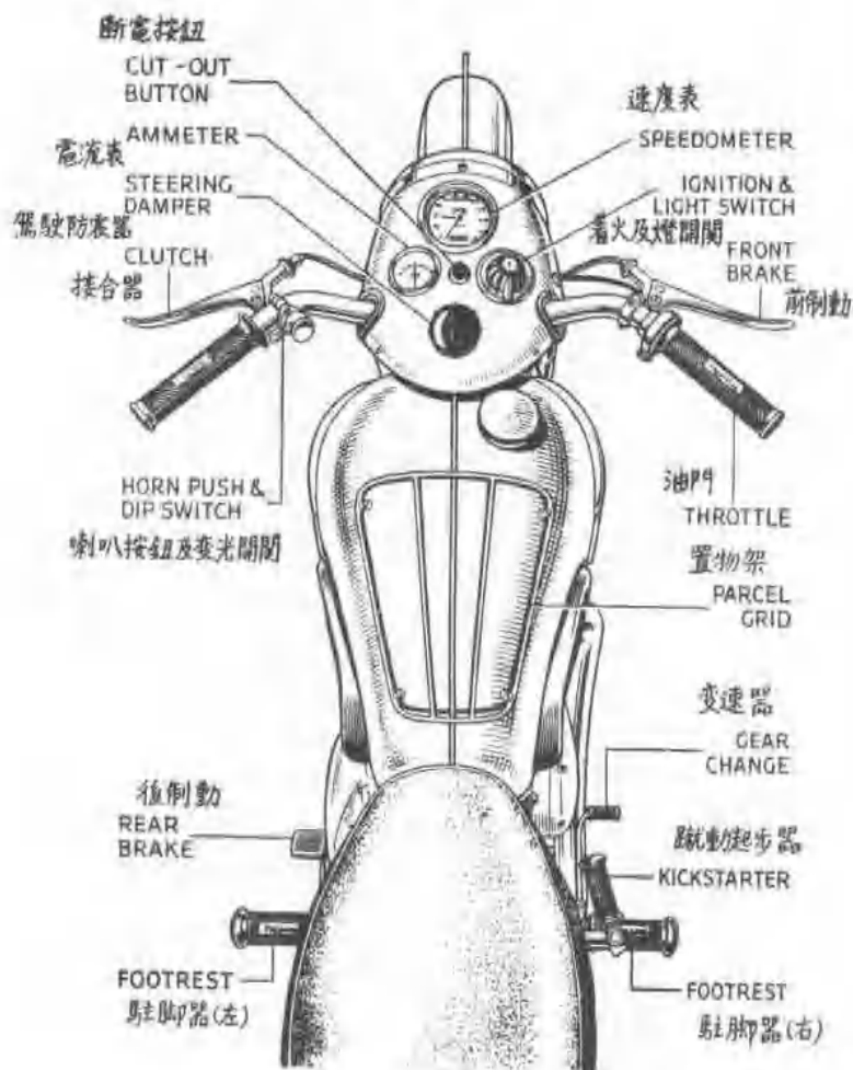
圖 5 一般電單車的操縱構件位置及說明
