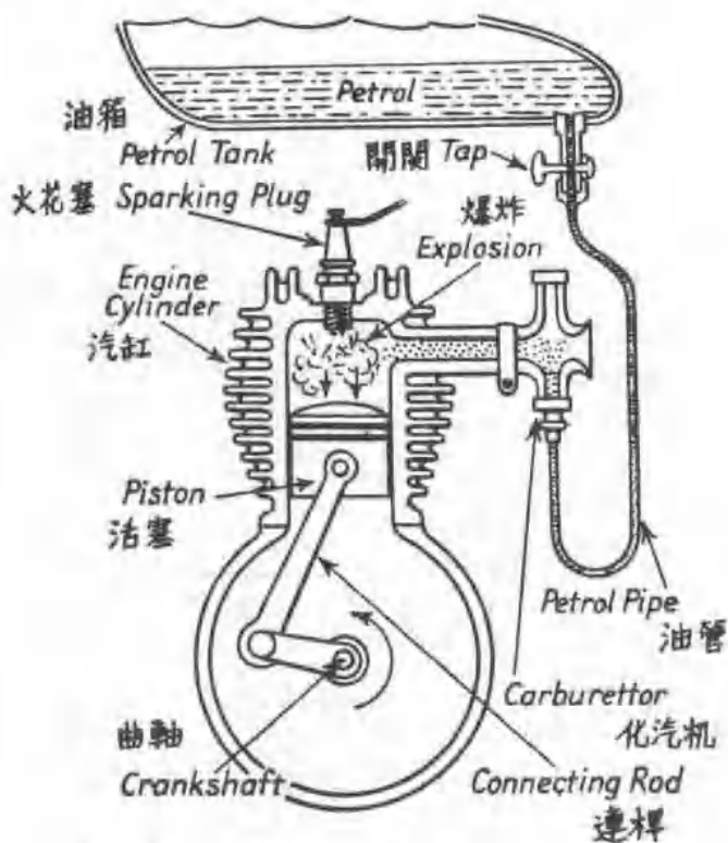
圖 6 電單車引擎的結構斷面，組零件及爆炸情形示意
