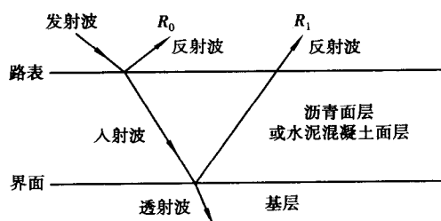
图 1.1.1 电磁波在路面面层中的反射
