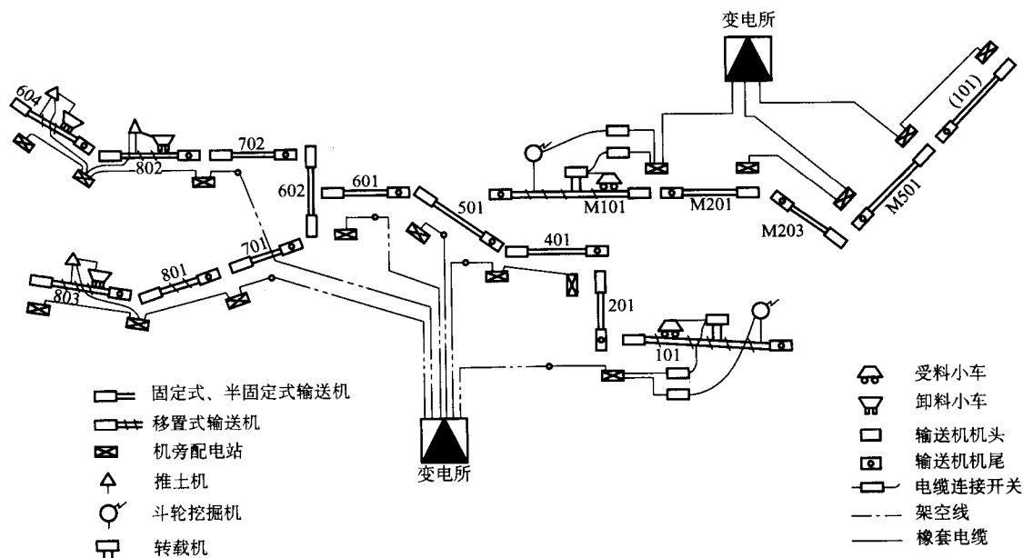
图 1-4 露天煤矿连续开采系统
