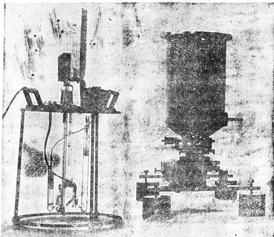
圖 1-1 由保護容器內取出之 \text{Kr}^{86} 光源。操作時以液態氮冷卻此燈。(英國 Teddington, 國立物理實驗室提供)。
