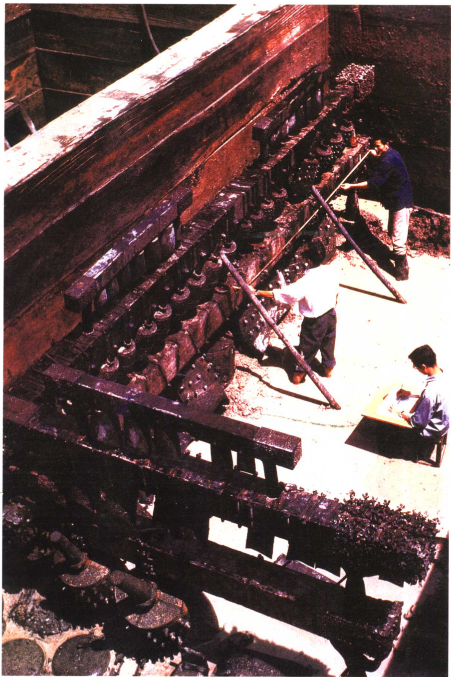
六 湖北战国曾侯乙墓地下音乐厅
