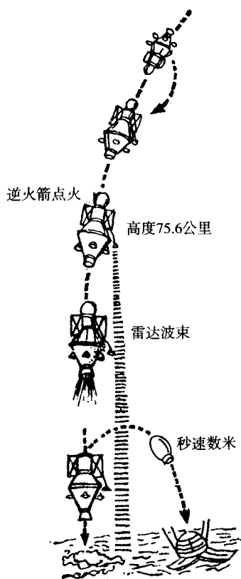
图 1.3.2 “月球”9 号软着陆方法
