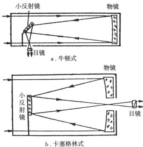
图 1.2.4 反射望远镜光路图
