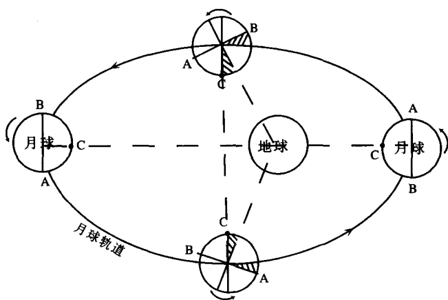
图 1.2.9 月球经度天平动
