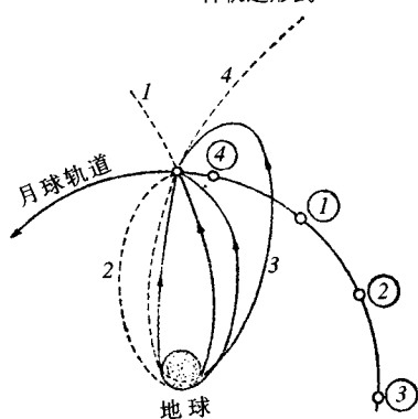
图 1.3.1 飞往月球的三种轨道形式
