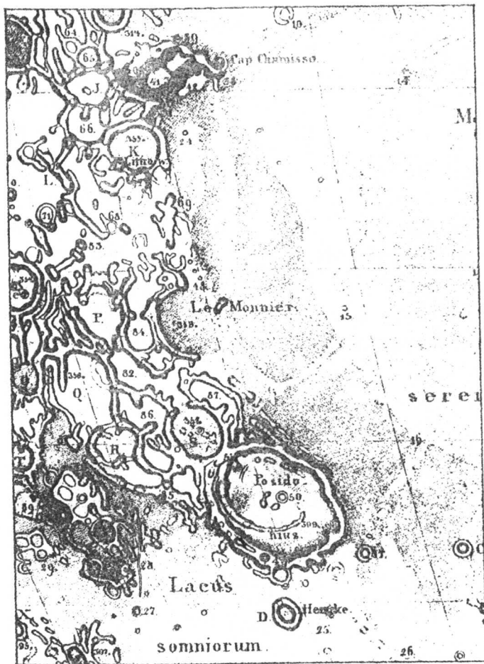
图 1.2.7 施密特于 1878 年出版的月面图之一
