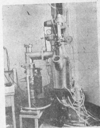
照片二 摄像机在单晶炉上的安装情况
