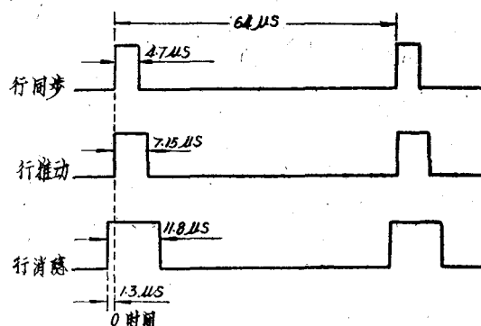
图十五 行同步波形
