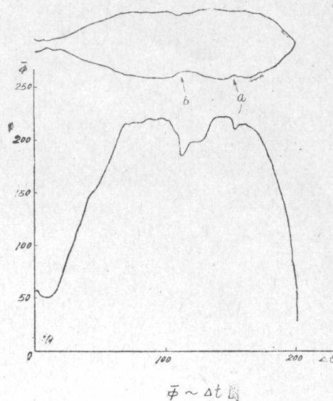
图十九 \bar{\phi} \sim \Delta t 曲线图
