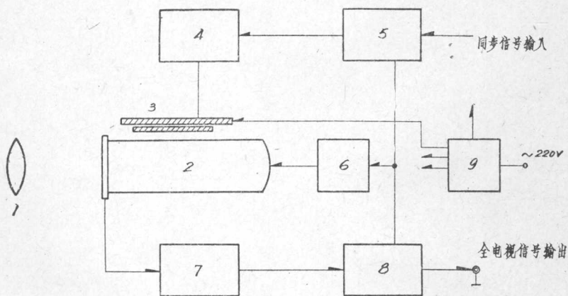
图七 摄像机的结构图
