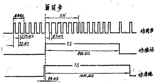
图十四 场同步波形
