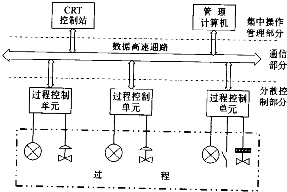
图 1-1 集散控制系统的基本结构
