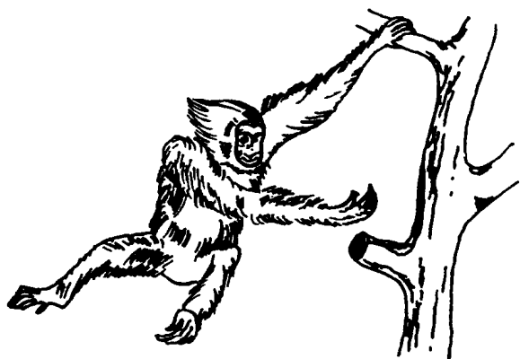
图3 长臂猿
