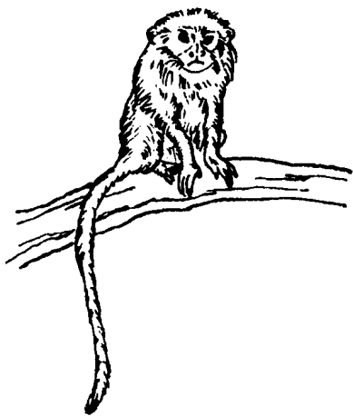
图 5 倭狨
