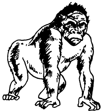
图 6 大猩猩
