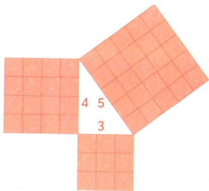
勾三股四弦五
