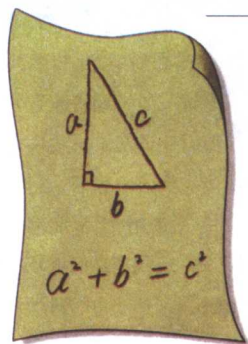
勾股定理
