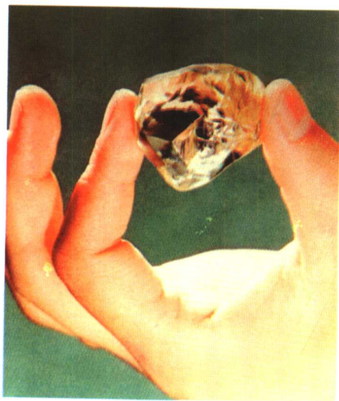
图版 23 常林钻石 (重 158.7860 克拉)
