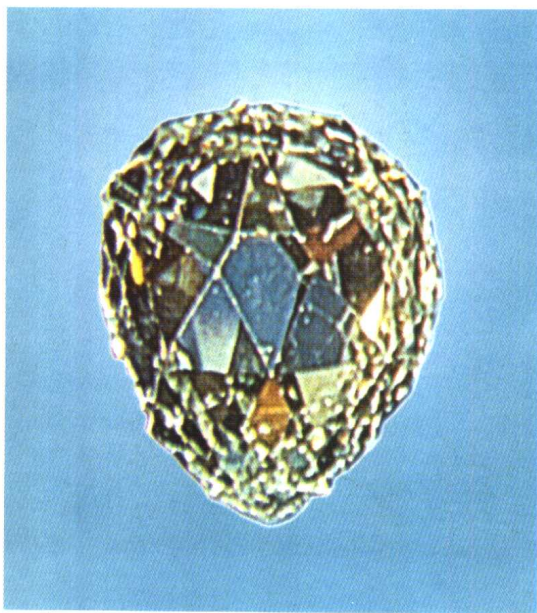
图版 8 桑西钻石(重 55 克拉)
