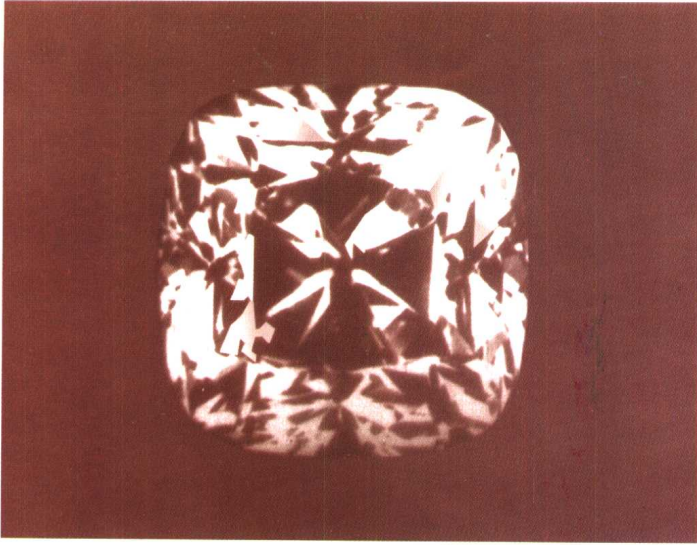
图版 3 红十字钻石(重 205.07 克拉)
