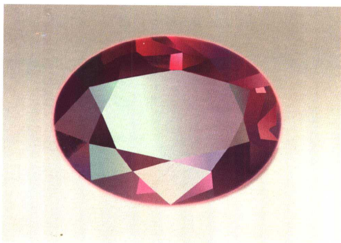
图版 21 变石(亦名亚历山大石)
