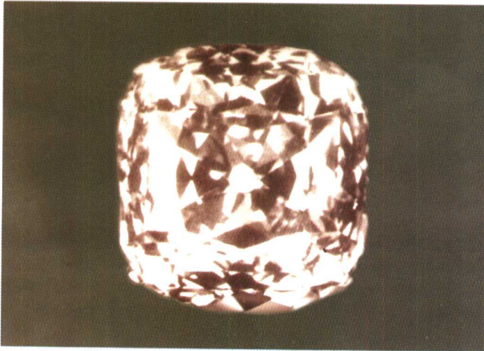
图版 4 塔菲尼钻石(重 128.51 克拉)
