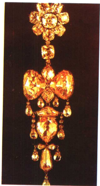
图版 9 马扎林钻石
