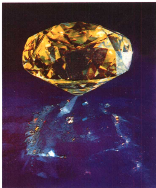
图版 12 德比尔斯金黄色钻石(重 234.65 克拉)
