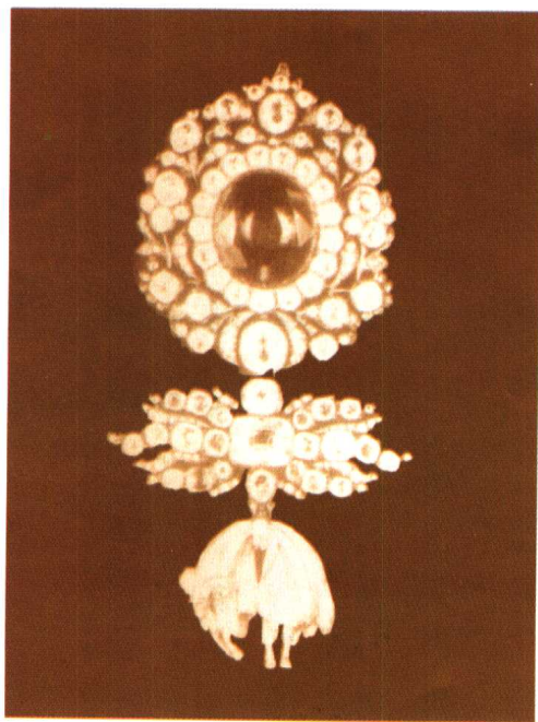
图版2 镶有韦特尔斯巴赫 钻石(重 35.32 克拉)的金羊 毛勋章
