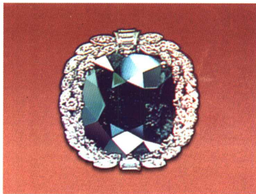
图版 13 黑色奥尔洛夫钻石(重 67.50 克拉)
