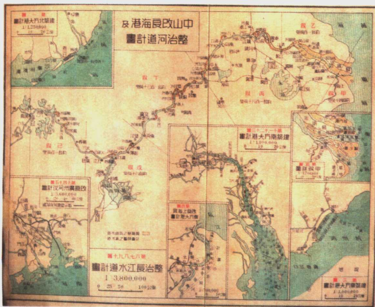
《中山改良海港及整治河道计划》（局部）
