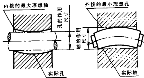
图 1—3 孔或轴的作用尺寸
