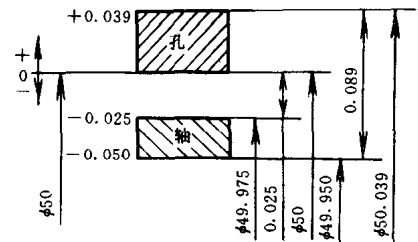
图 1—6 间隙配合公差带
