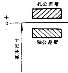
图 1—2 公差带图
