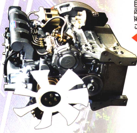
SL系列三缸柴油机
