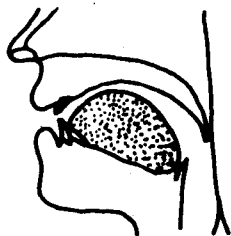
[i] 的口腔示意图
