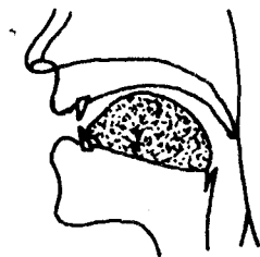
音素 [i:] 的口腔和唇形图
