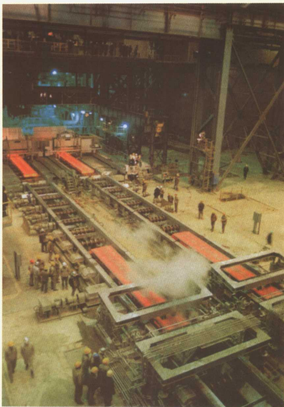
上海宝山钢铁集团公司连铸车间
