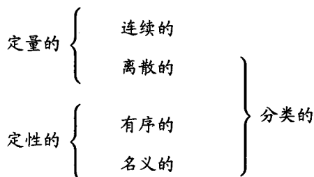
图 1.1-1 变量的类型
