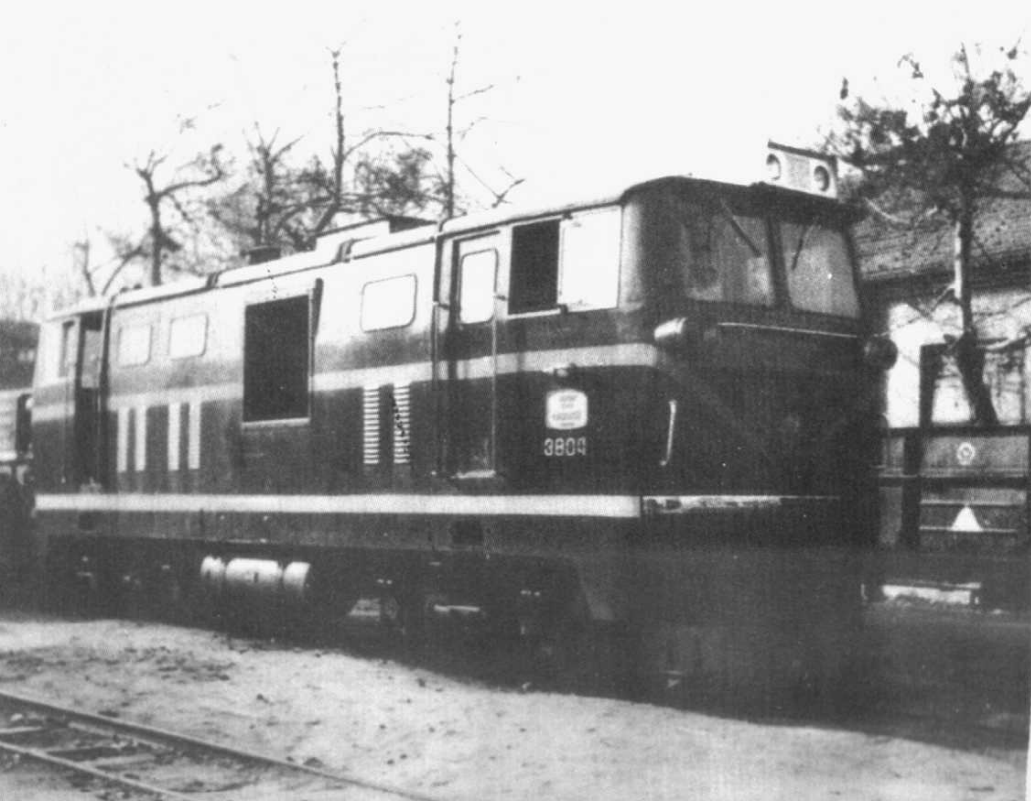
地方铁路内燃机车
