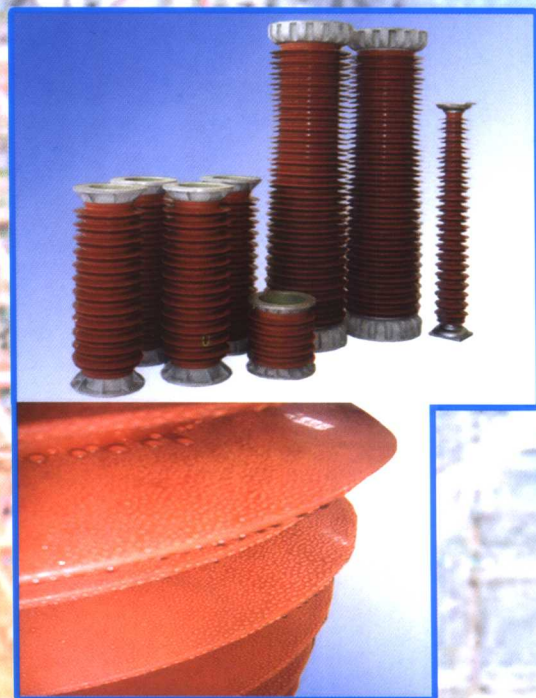
空心绝缘子
