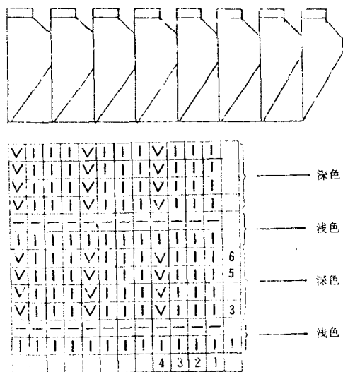
图 1-1 帽型起片及针法编织图
