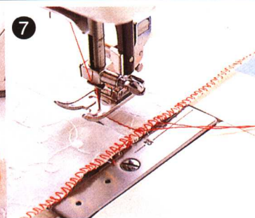
缝左侧缝线的松紧带通口。
