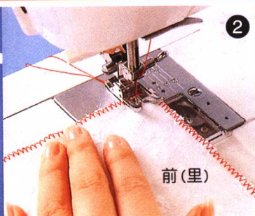
前后片面对面从距布边 1cm 内侧开始缝。
