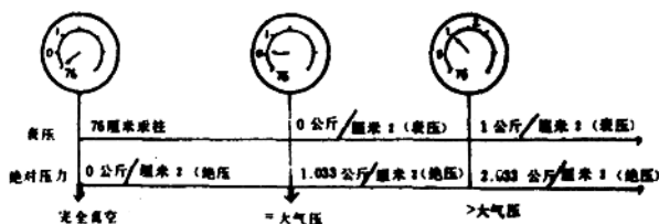
图 1-3 绝对压力和表压之间的关系
