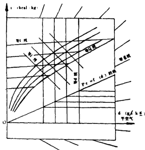
图 1—7 空气 i—d 图
