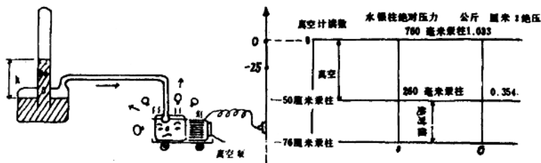
图 1-4 真空度
