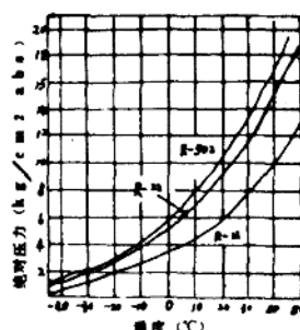
图 1-6 几种制冷剂的饱和温度与压力曲线
