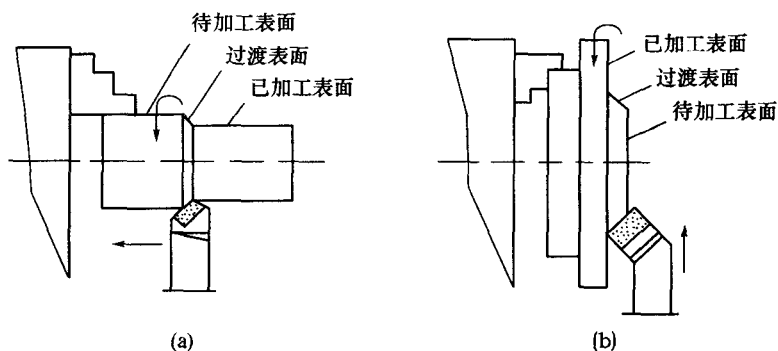
图 1-2 工件上的加工表面
