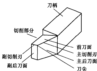
图 1-3 刀具切削部分结构要素
