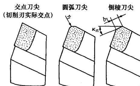
图 1-4 刀尖形状
