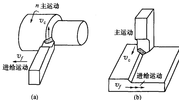
图 1-1 主运动与进给运动 (a) 车外圆; (b) 刨平面。
