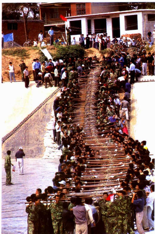
2002年9月4日，千余军民共建洹河橡胶坝
