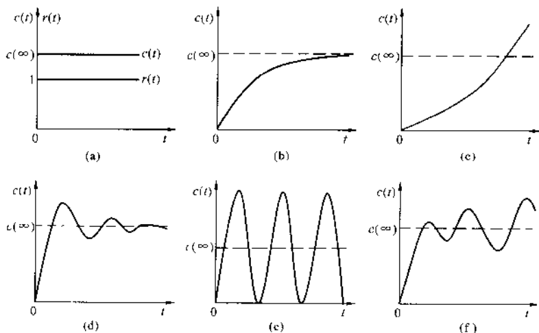
图 1-9 系统单位阶跃响应曲线
