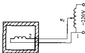
图 1-3 炉温开环控制系统
