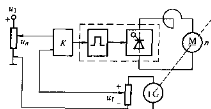
图 1-5 闭环调速系统
