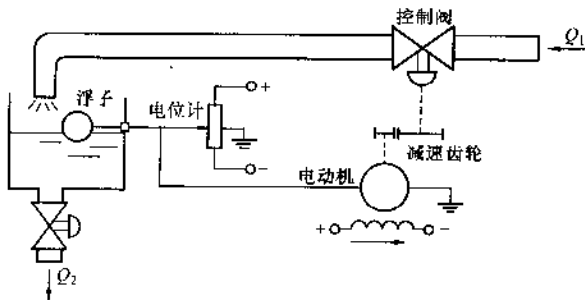
图 1-11 习题 1-6 的液位自动控制系统的示意图
