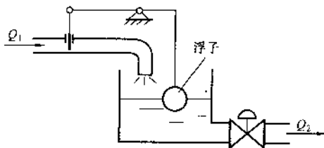
图 1-10 习题 1-5 的水位自动控制系统示意图
