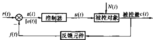
图 1-8 简化的闭环系统组成方框图
