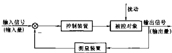
图 1-4 闭环控制示意图
