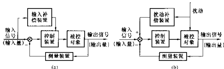
图 1-6 复合控制示意图
