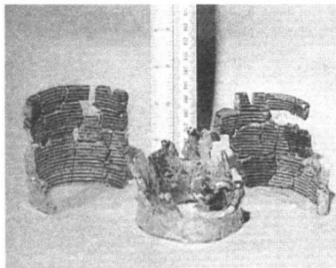
被炸裂的钢管
