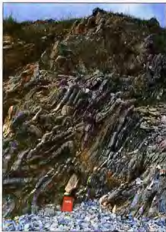
内力作用使岩层发生褶皱
