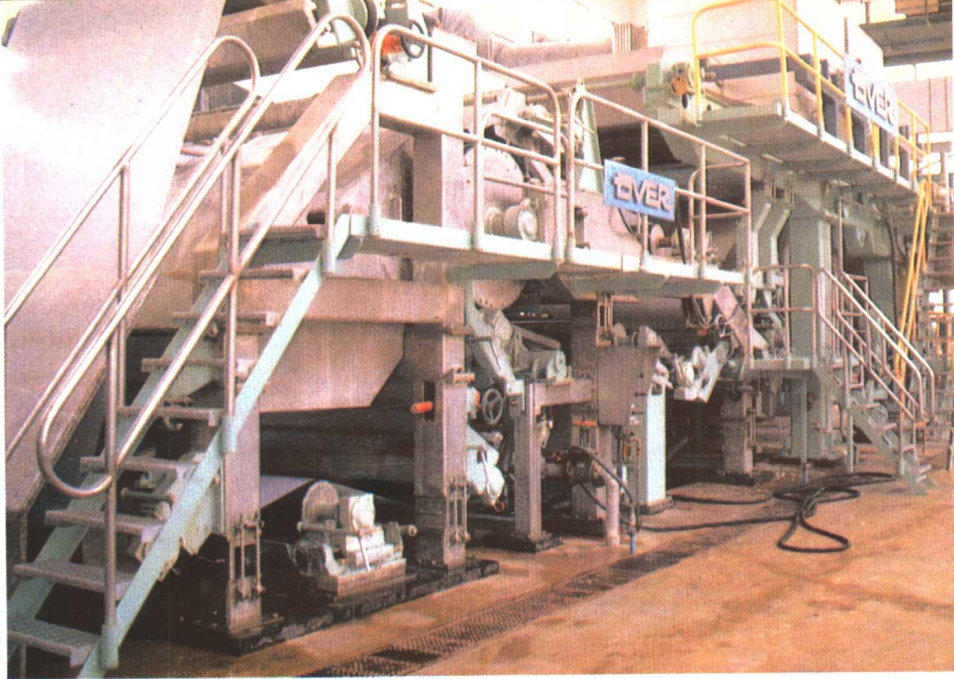
◀ 连云港造纸厂夹网卫生纸机
