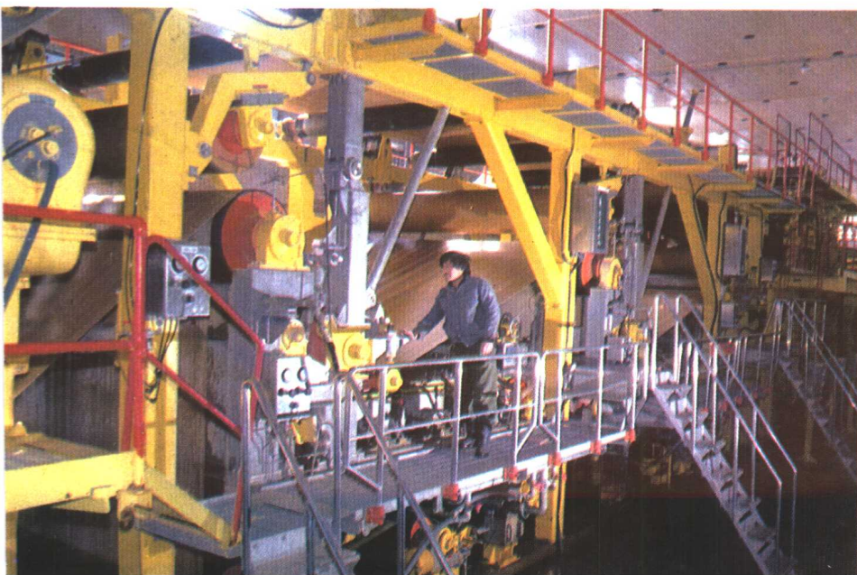
◀ 营口造纸厂1989年 建成年产4万吨涂 料白板机的新型 成形网部
