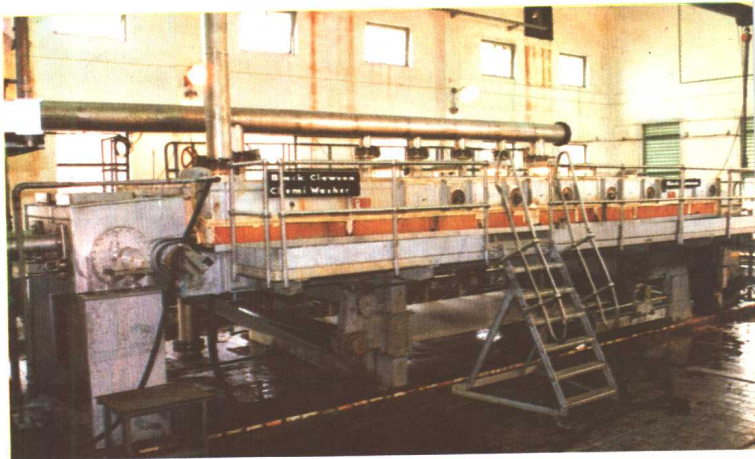
▲广州造纸厂带式洗浆机
