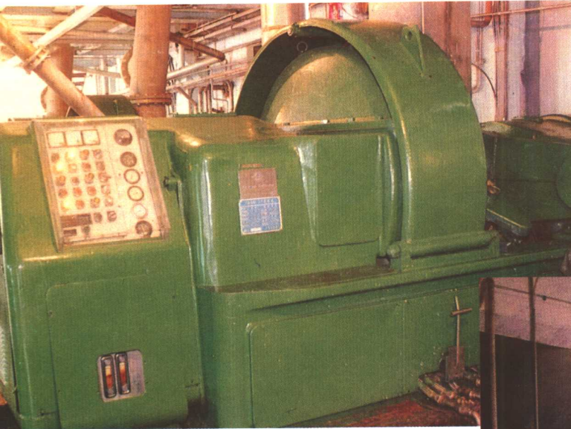
▲吉林造纸厂CTMP化机浆盘磨机
