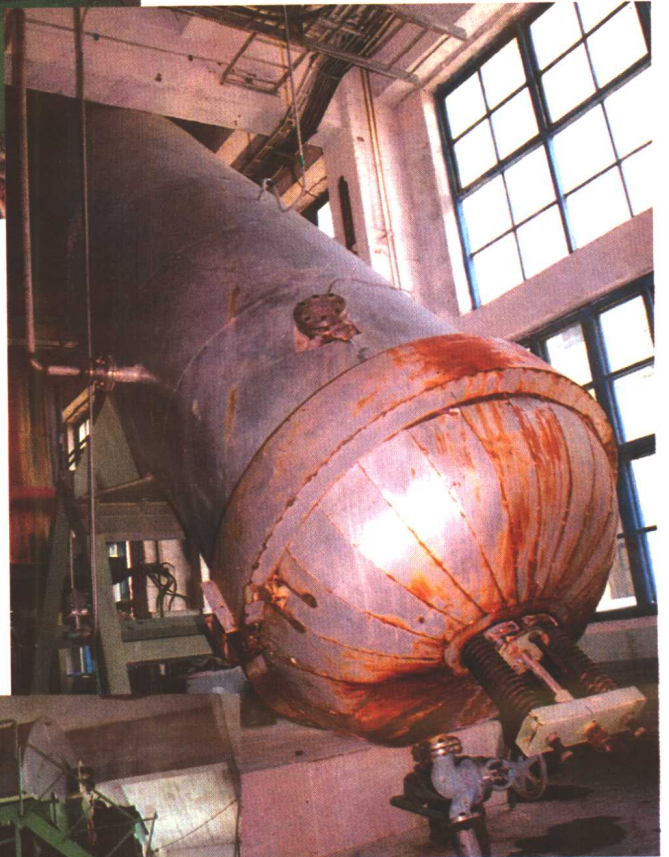
▶石岘造纸厂SCMP系统M&D连续蒸煮器
