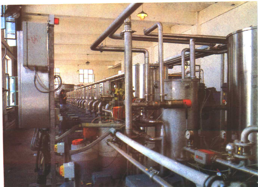
▶开山屯化学纤维浆厂 红液超精滤设备
