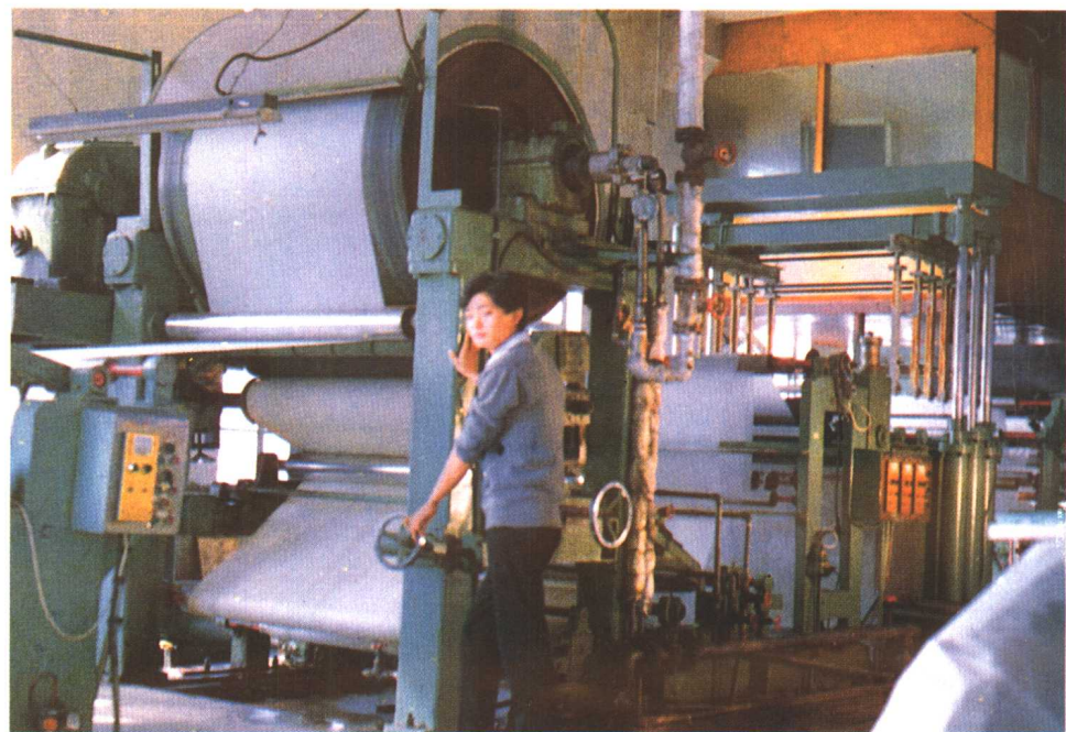
▶ 杭州新华造纸厂茶叶袋纸机
