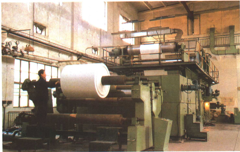
▶ 山东造纸总厂西厂 玻璃卡纸铸涂机
