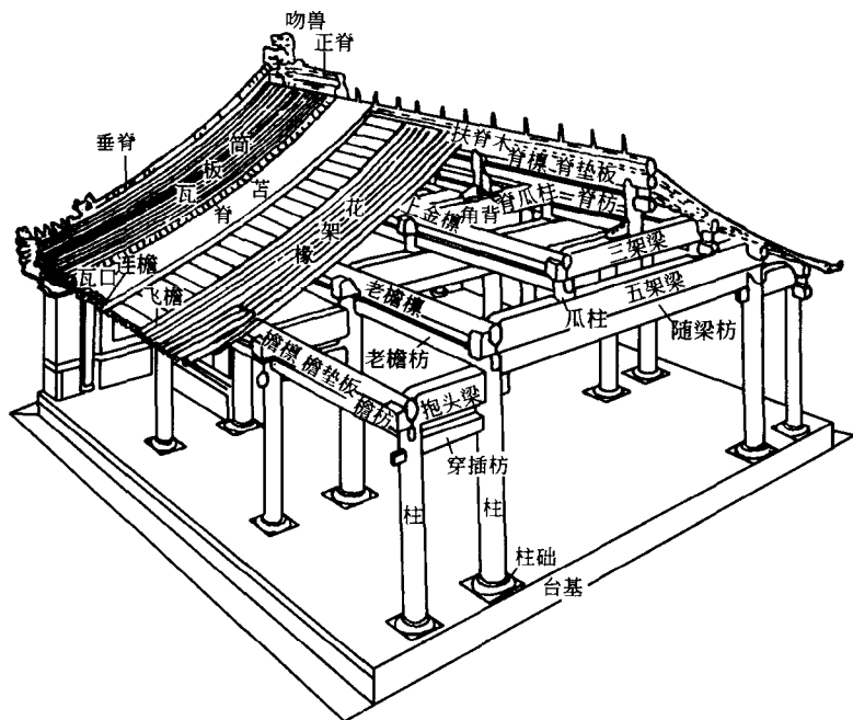
图 1-1 叠梁式木构架
