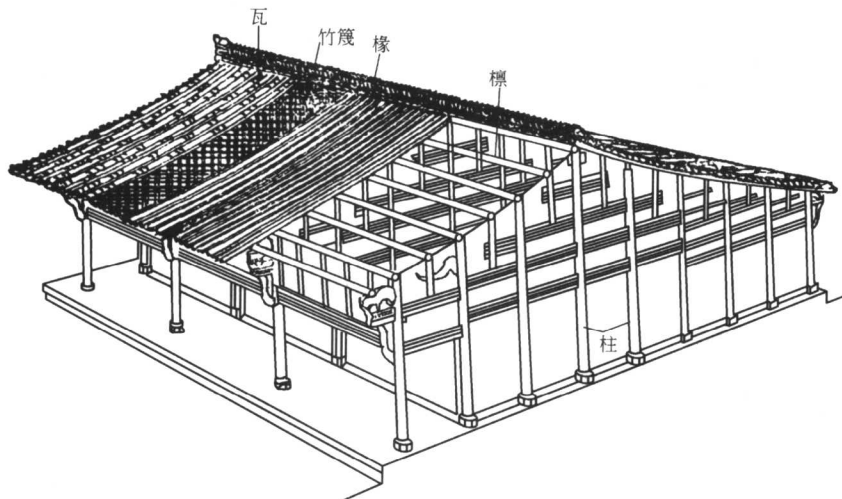
图 1-2 穿斗式木构架
