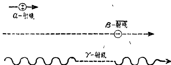
圖2. α射綫能貫穿空氣達10公分 β射綫能貫穿空氣達20公尺 γ射綫能貫穿空氣達數百公尺
