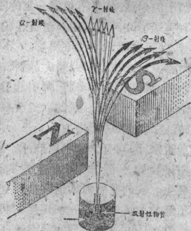
圖1. 放射性物質放出來的射線，在強有力的磁極之間，被分裂成爲向左、向前和向右的三種射線，這就是 \alpha 射線（又叫甲種射線）、 \beta 射線（又叫乙種射線）和 \gamma 射線（又叫丙種射線）
