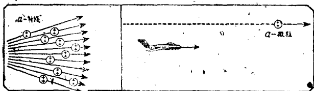
圖 3. \alpha 射綫是由運動極為迅速的帶正電荷的質點組成，它的速率每秒鐘 20,000 公里，比現代噴氣式飛機快 7 萬多倍。
