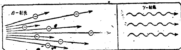
圖 4. \beta 射線本是些電子（負電荷），速度每秒鐘 200,000 公里。 \gamma 射線是一種波長很短的電磁波，每秒鐘的速度和光速相同（300,000 公里）。
