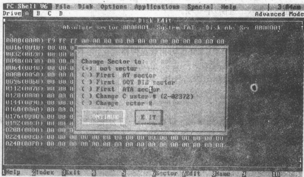
图 1-2 PCSHELL 中显示扇区位置的选择
