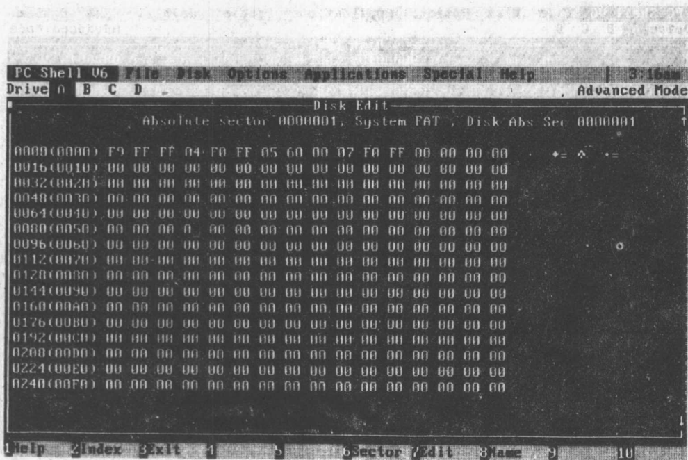
图 1-4 新的 EDIT.COM 文件的 FAT 表
