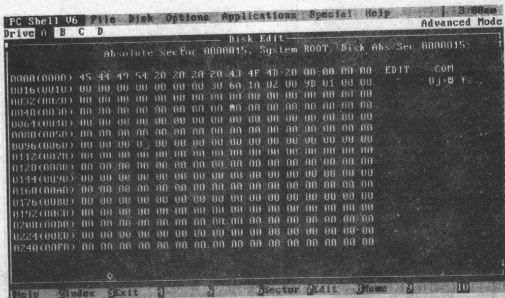
图 1-3 A 盘存有文件 EDIT.COM 后的 ROOT 表
