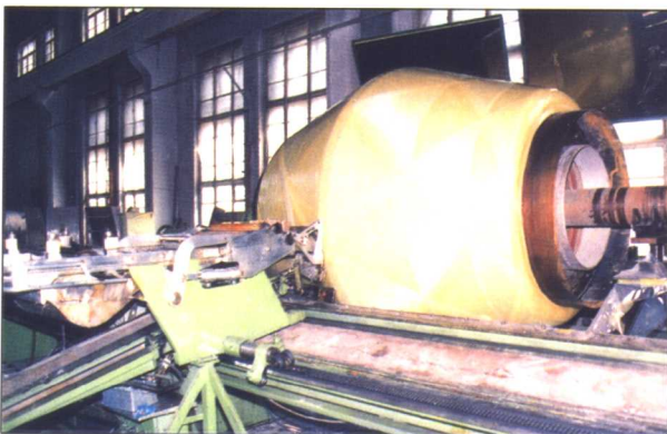
制造中的 60 万千瓦发电机组玻璃钢定子锥壳
